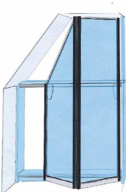
Obr.5. Vrchná koľajnica je montovaná na policu.
